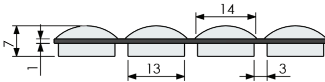
Perçin Birleştirmeli Al. Palet - ALP3 (Bombeli)
